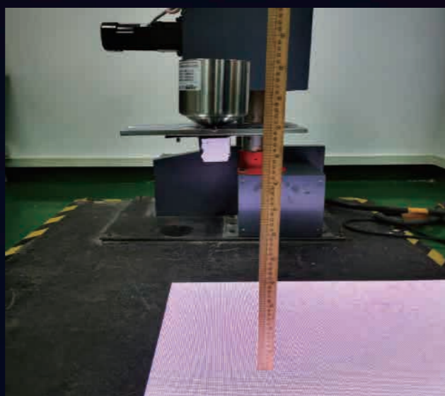
坠落测试 1k10
